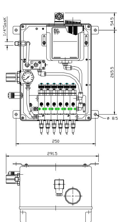
AFMETINGEN UCGF - SE
