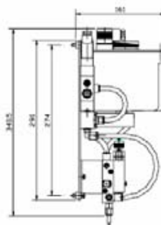
ENCOMBREMENTS AGGF
