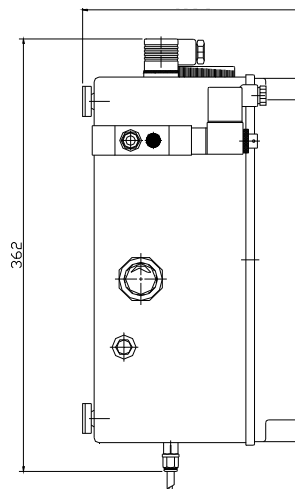
DIMENSIONS UCSG
