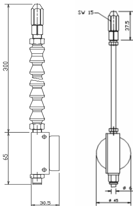
Code 70.100.2 FLEXIBEL LOCLINE MET MAGNEET FLEXIBEL LOCLINE AVEC AIMANT
