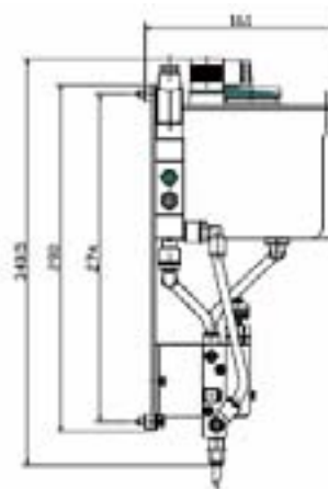
ENCOMBREMENTS AGSG
