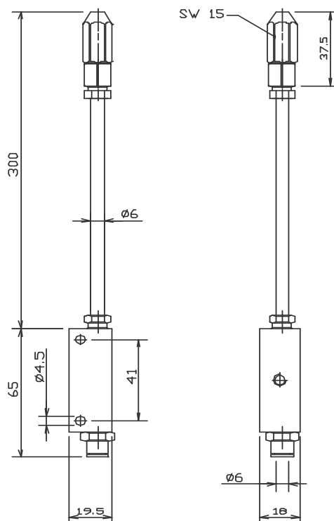
Code 70.100.1 SPROEIER VAST ZONDER MAGNEET PULVERISATEUR FIXE SANS AIMANT
