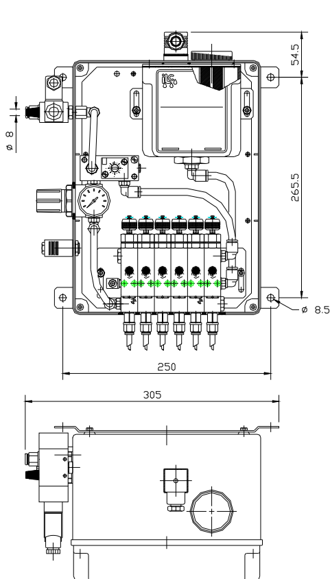
AFMETINGEN UCGF
